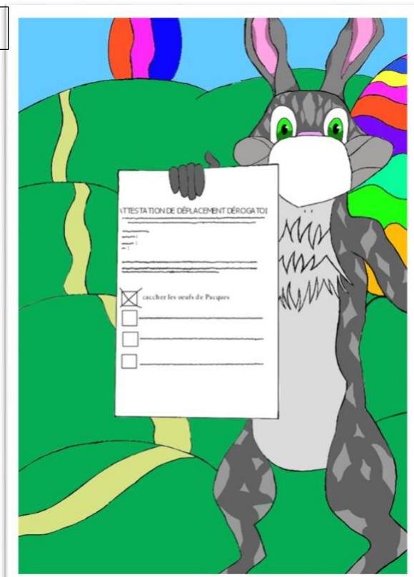
Dylan Novo
